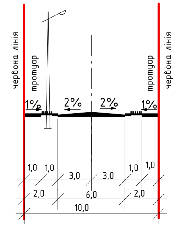
Креслення поперечних профілів вулиць М 1:200 Житлові вулиці
